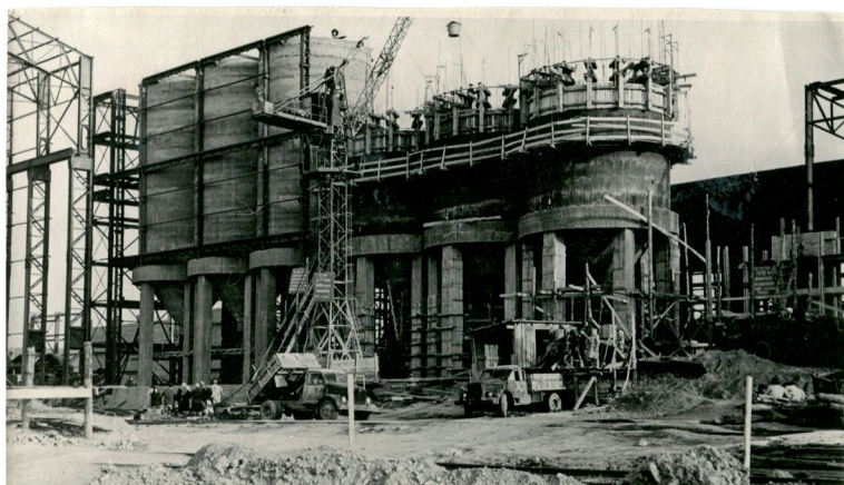
Строительство вертикальных бассейнов Алексеевского цементного завода. Конец 1950-х гг.
